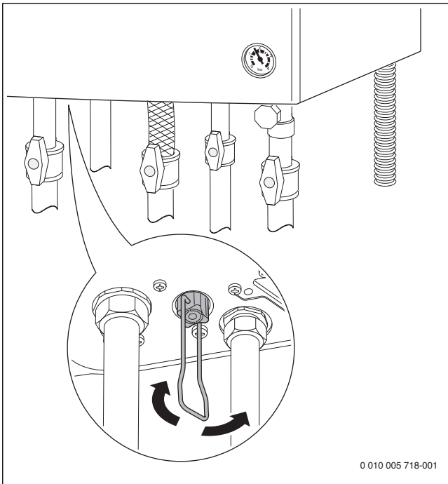
Мал. 4 Кран для заповнення опалювальної установки
